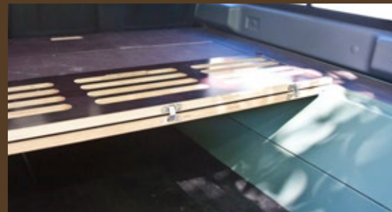
Klappbare Laderaumabdeckung
